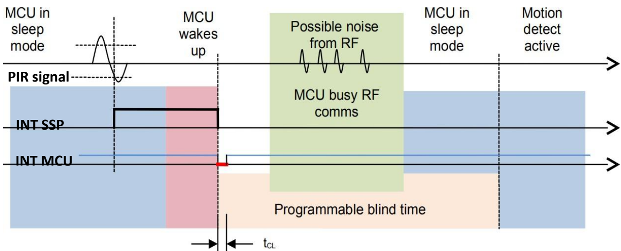
运动检测及触发清除时序图
