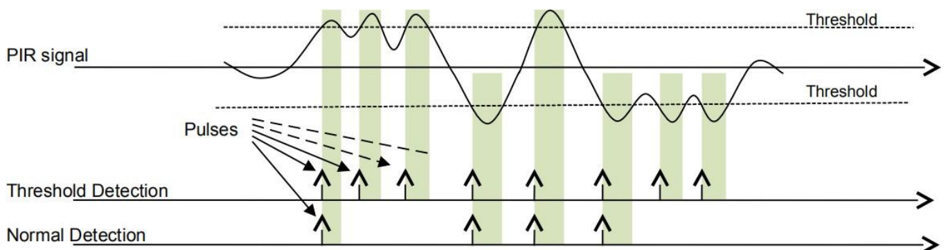
运动检测脉冲计量算法的两种模式
