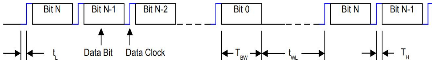
SERIN输入接口的控制时序图
