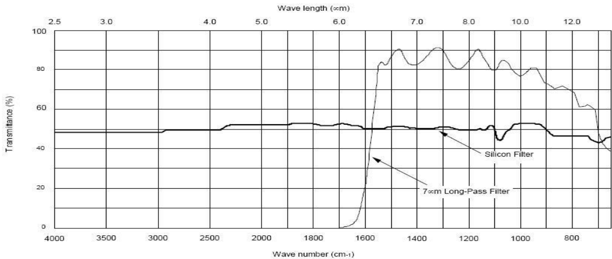
滤光片光谱特性
