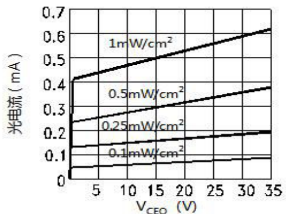
图六：光电流VS V_{CE0} 曲线
