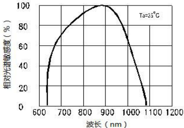
图一：光谱敏感度曲线
