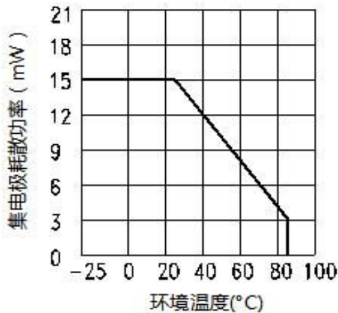
图三：耗散功率VS环境温度曲线
