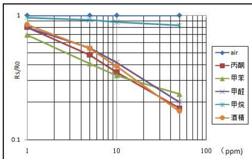
不同气体灵敏度曲线对比
