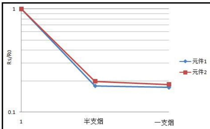
元件在18L气箱中测试自然燃烧香烟所得灵敏度曲线
