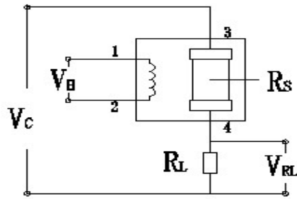
图2： MP135A 测试电路
